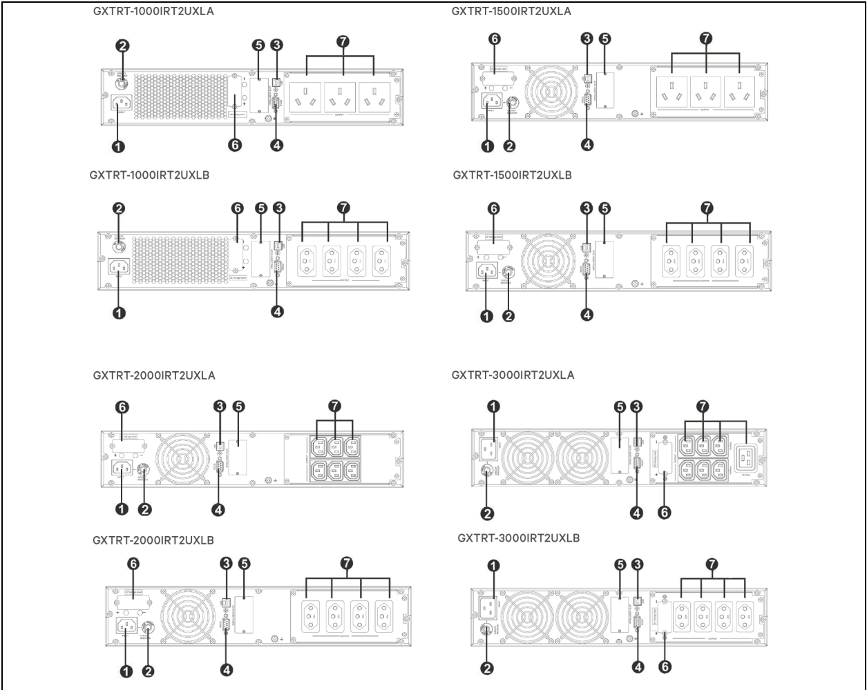
Figura 2.1 Painéis traseiros
